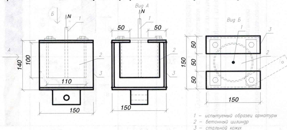
Рис. 1. Схема захвата испытуемого образца
