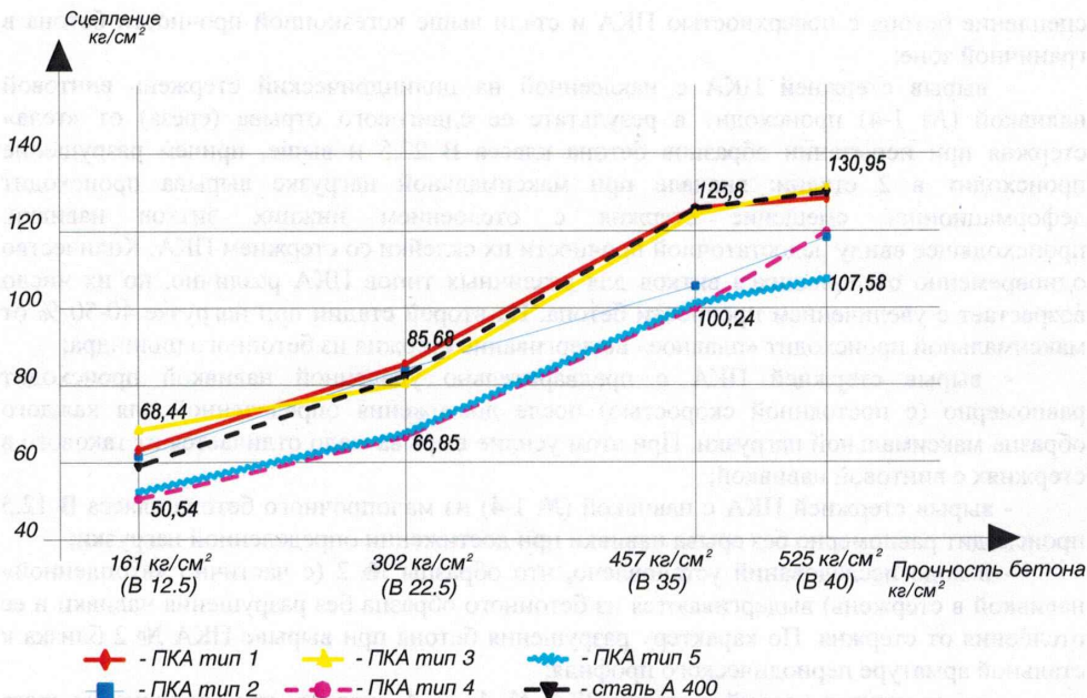
Рис. 2. Прочность сцепления различных типов ПКА и стали с бетоном различной прочности
